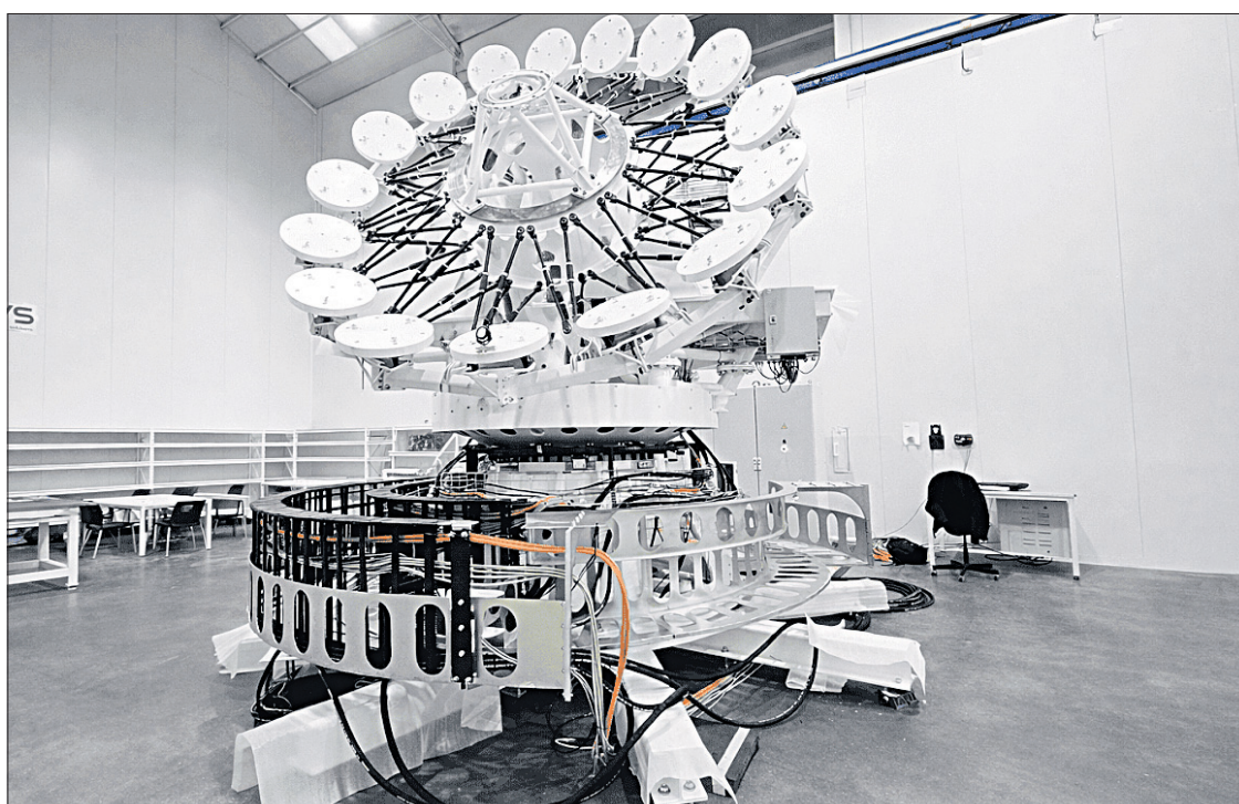
▲ Estructura principal del telescopio SELF. Foto tomada de la página del IAC
